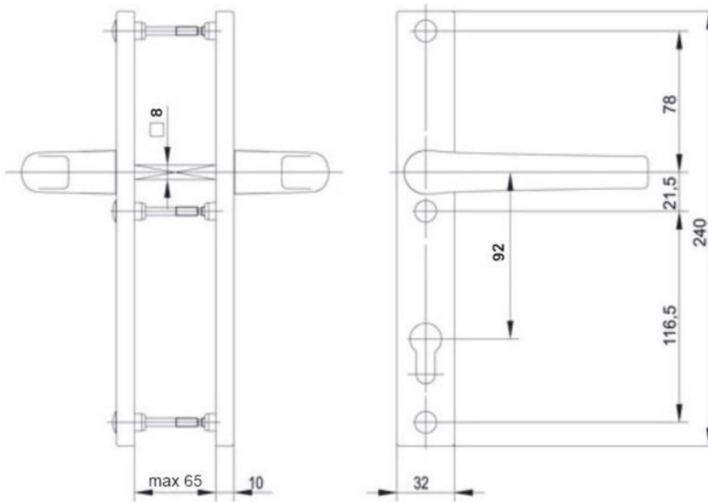
Rysunek: Wymiary Klamki
